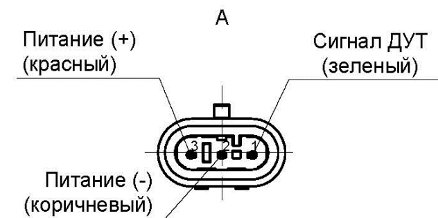
Рисунок 1 - Назначение выводов разъема подключения ДУТ.ТИТАН.А
